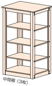
中間棚(3枚)
